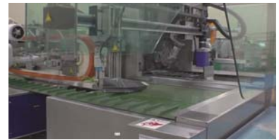
年間を通して 15℃、集塵装置も完備した、人にも花にもやさしい花加工場
